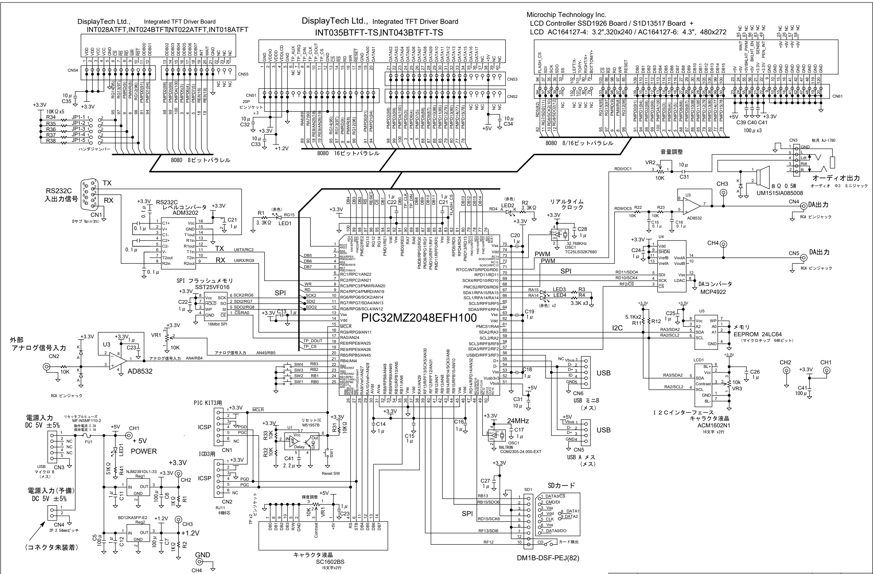
PIC32MZ評価ボード電気回路図 (汎用モジュール評価ボード DB001搭載)
